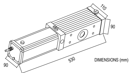
12710800 Spar for SCUTI 1,75 m (n. 2 pcs) adjustable with several fixing holes Longherone per SCUTI 1,75 m (n. 2 pz) regolabile con molteplici fori di fissaggio
